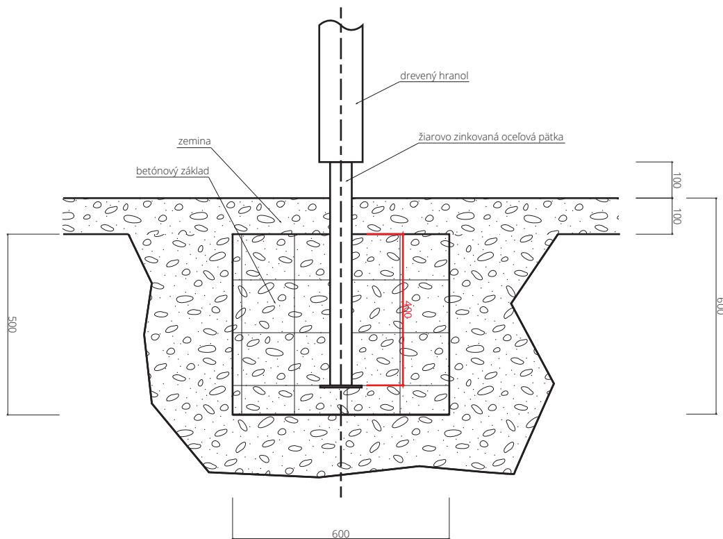
Detail ukotvenia
